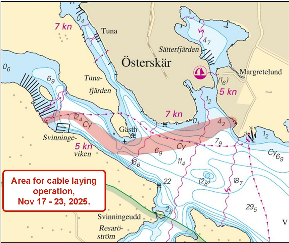
Förläggning av sjökabel S om Gästholmen och Österskär
