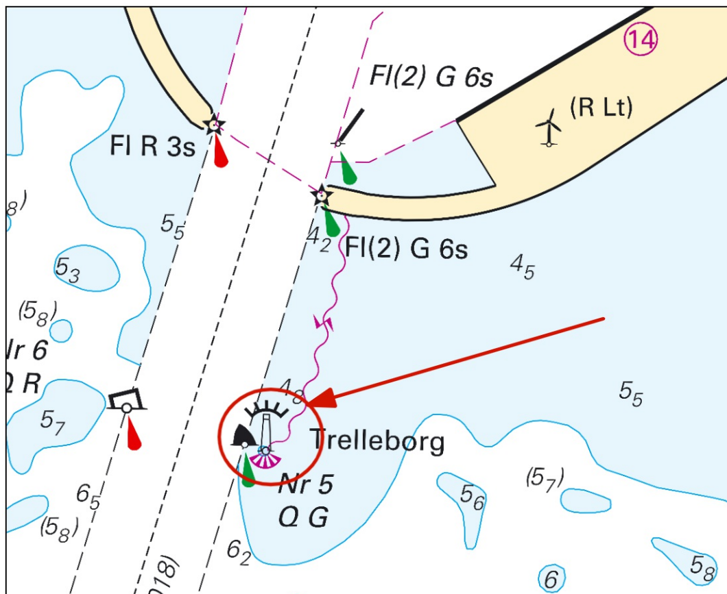
Radarreflektor
