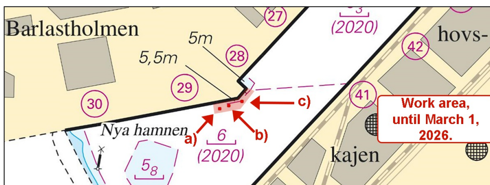
Arbetsområde och positioner för prickar vid Barlastholmen
