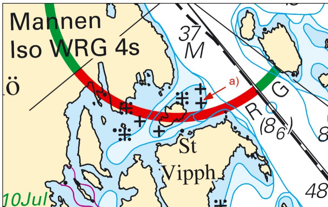
Undervattenssten med förändrad djupkurva
