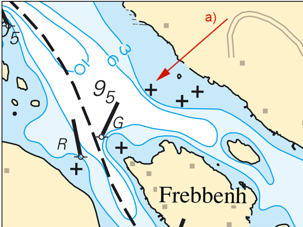
Undervattenssten och utökad 0-3 m djupkurva, Frebbenholmen.
