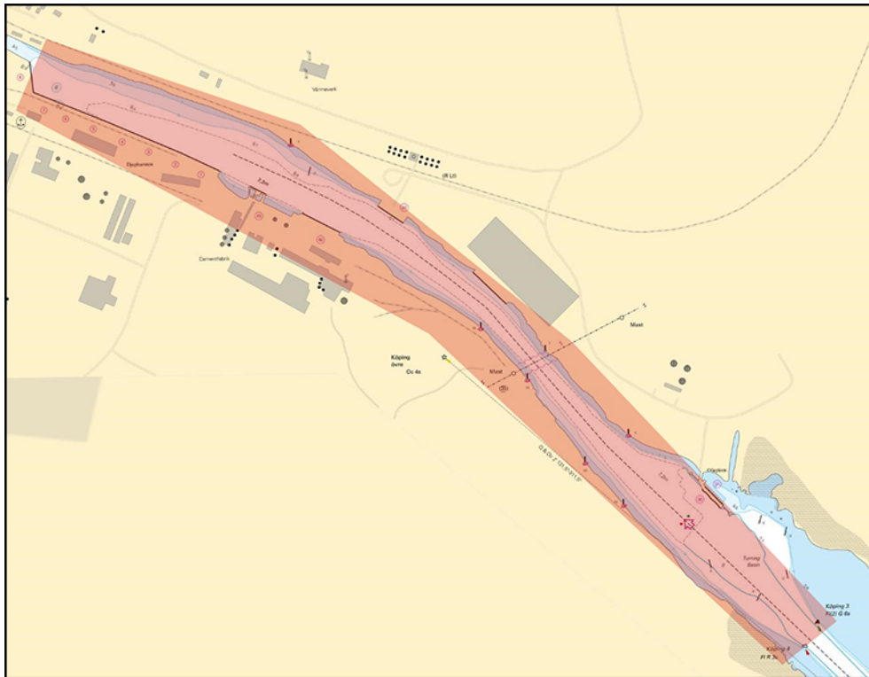
Köpings hamn, område där muddring pågår.
