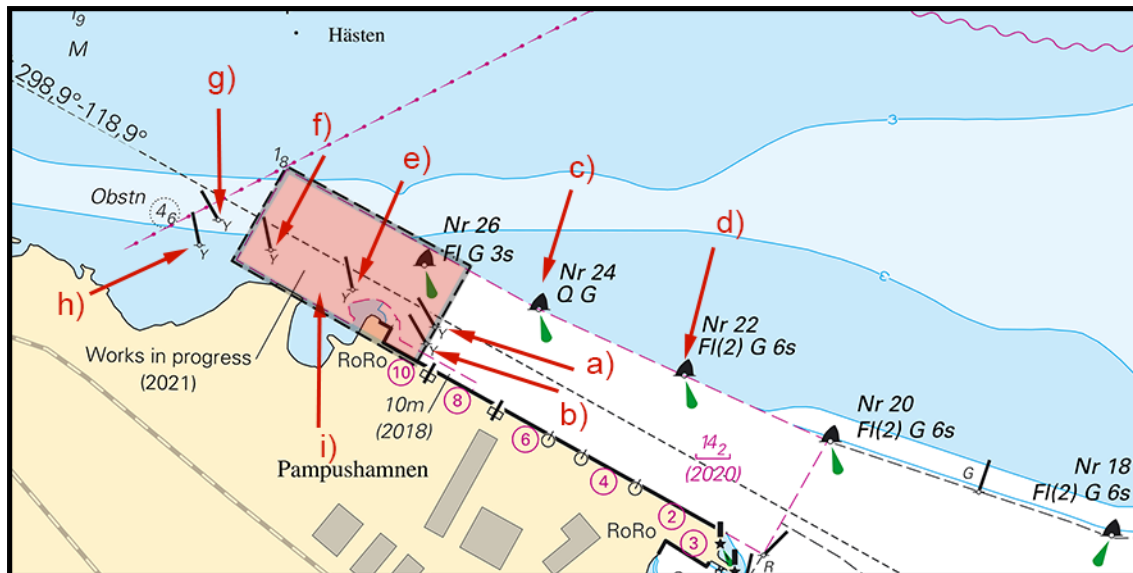
Pampushamnen, Norrköping. Ny utmärkning.
