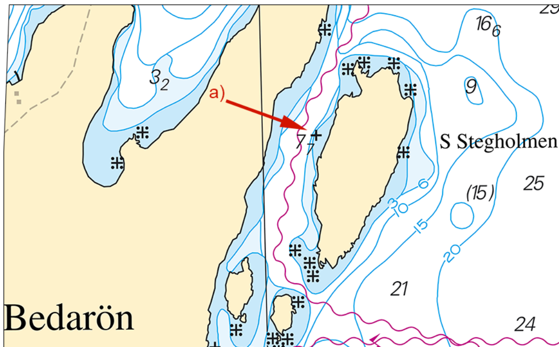
S Stegsholmen, undervattenssten och justerad djupkurva.
