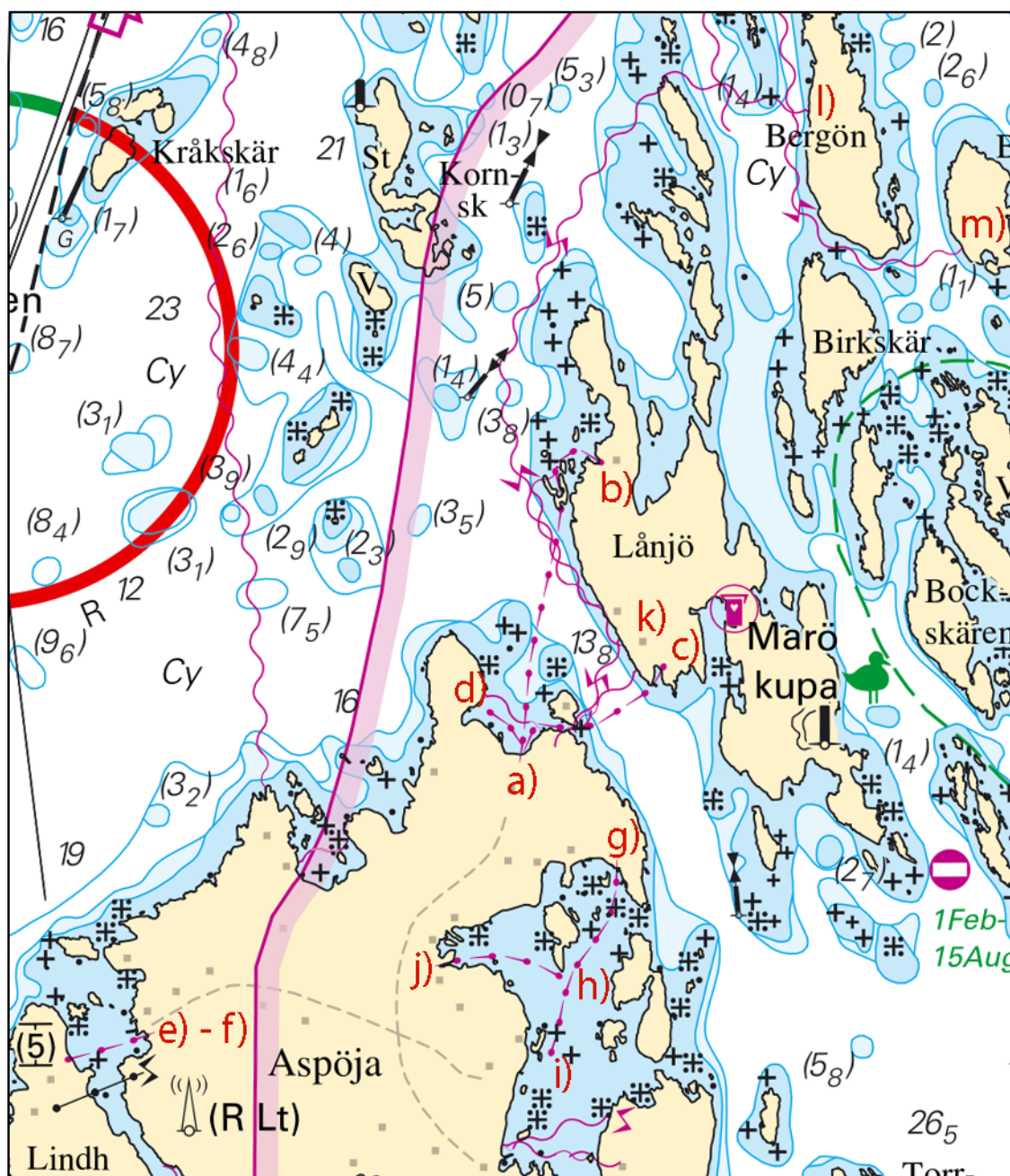
Aspöja. Rörledningar och sjökablar, el
