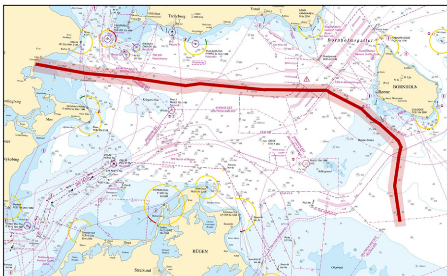
Undersökningskorridor - Baltic Pipe
