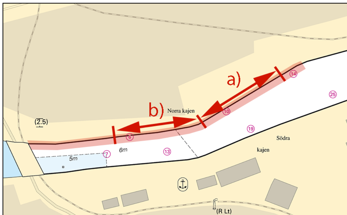
Norrköping. Inre hamnen. Norra kajen. Ombyggnadsarbeten
