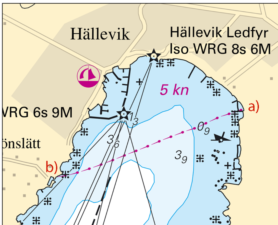
Hälleviksbukten, rörledning
