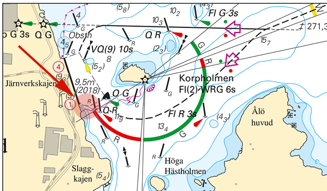
Dyk- och sprängningsarbeten vid Järnverkskajen, Oxelösund
