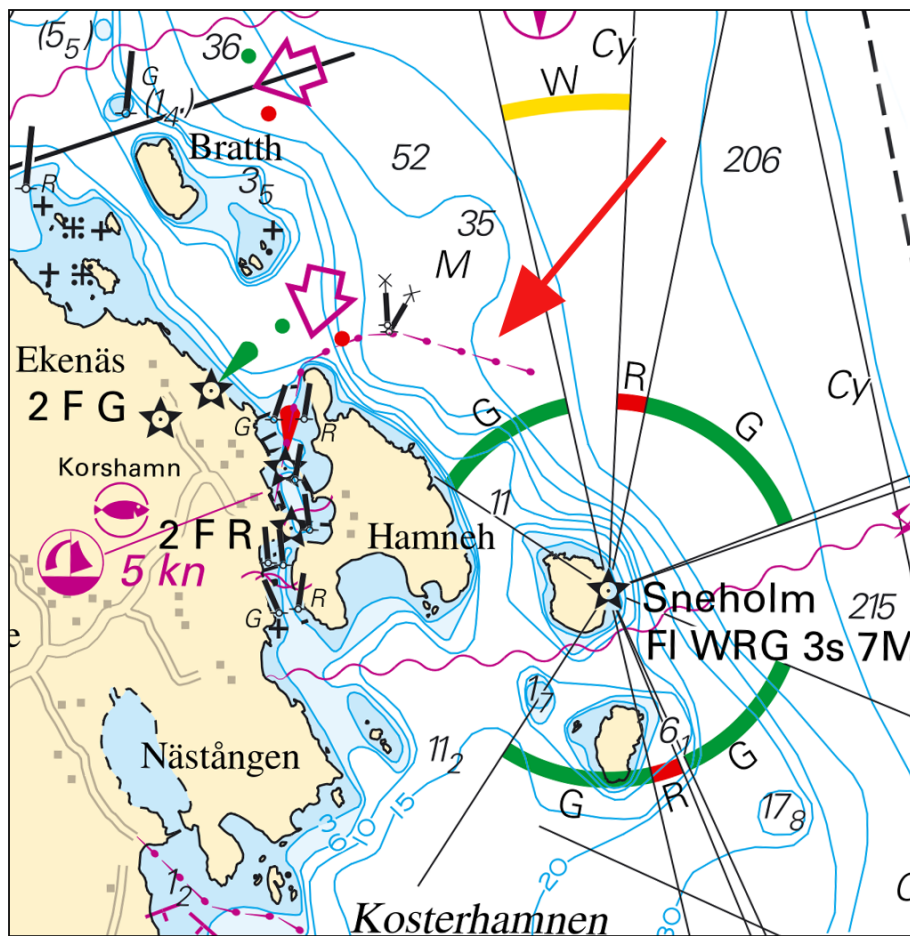
Förläggning av rörledning
