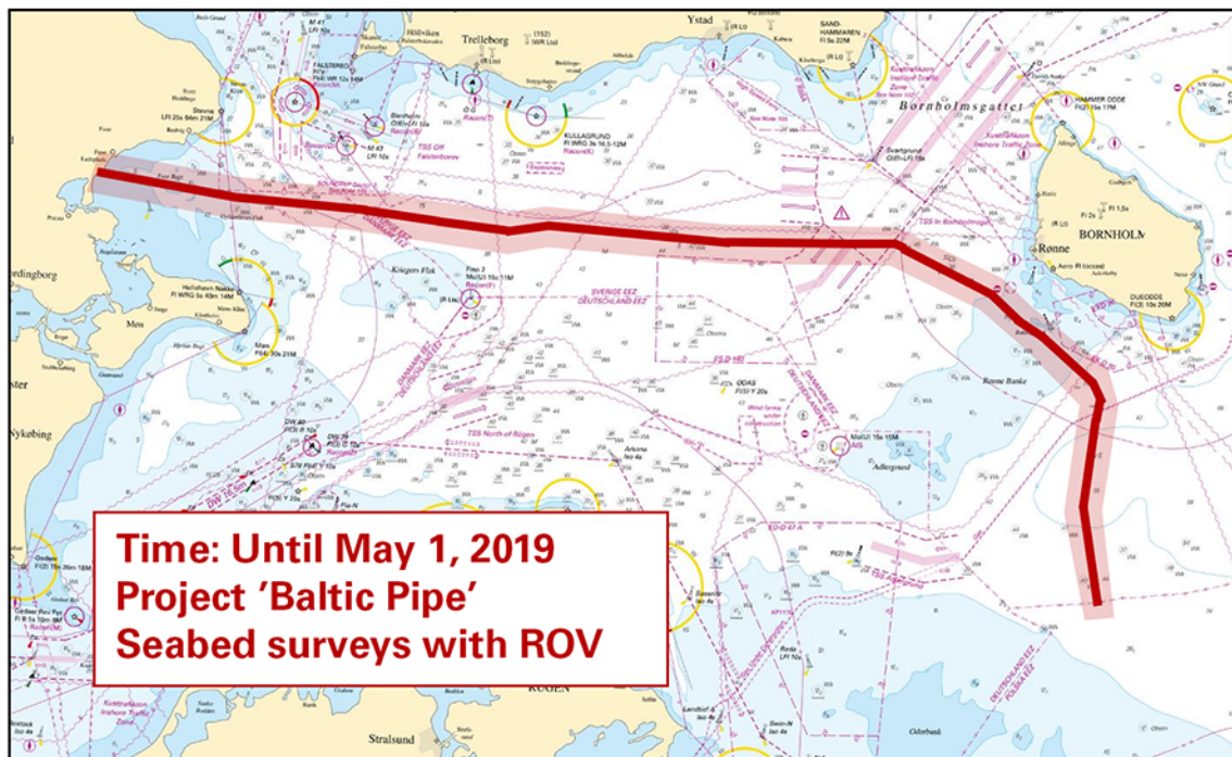
ROV undersökningar, Baltic Pipe Project
