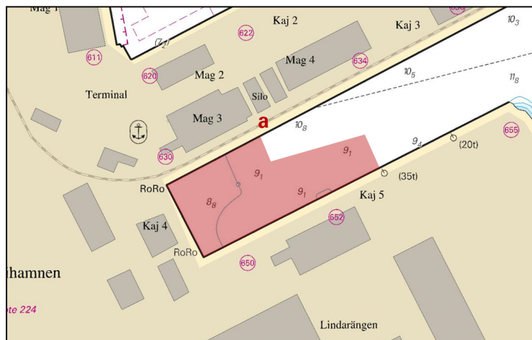
Muddringsområde - Frihamnsbassängen
