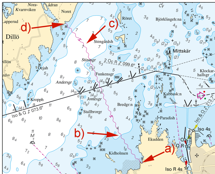
Sjökabel, Mariestad - Torsö
