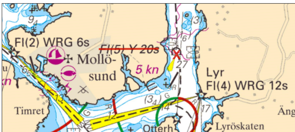
Tångesund, lysboj indragen
