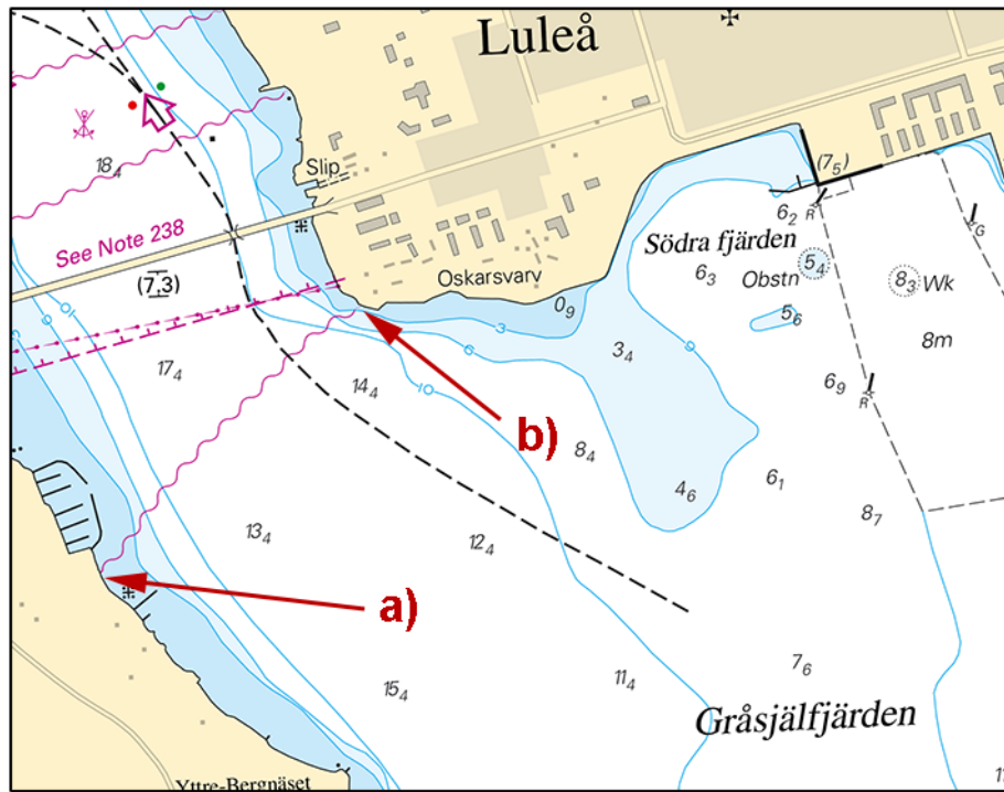
Sjökabel i Luleå
