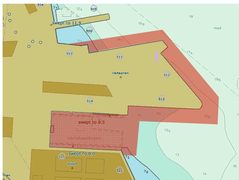
Sjömätning i Värtahamnen
