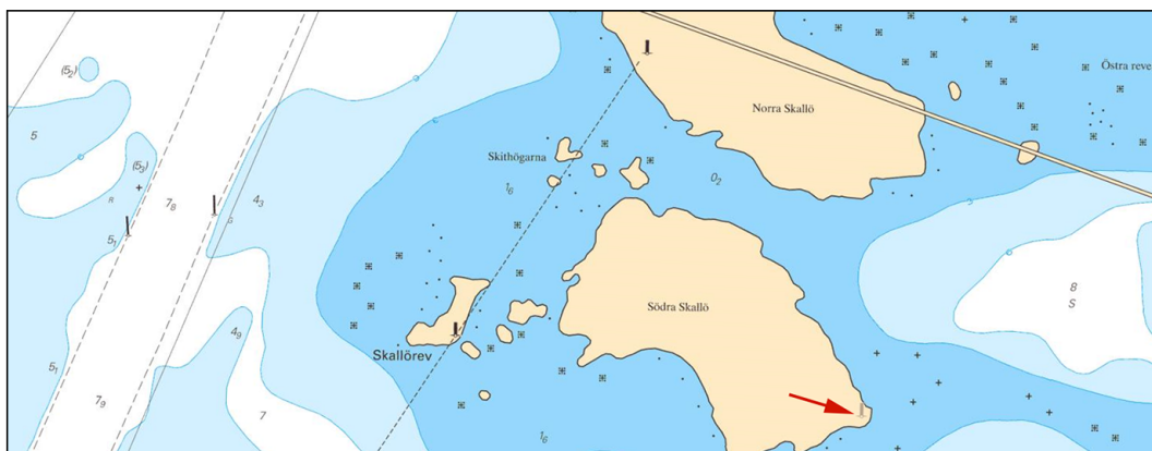
Sjömärke på Södra Skallö avlägsnat
