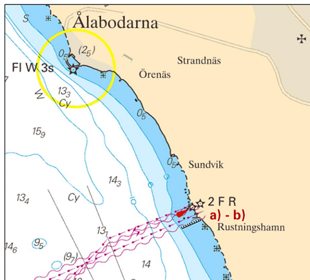
Fasta fiskeredskap S om Sundvik
