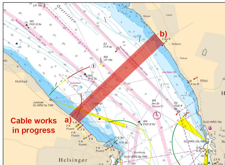
Kabelarbeten i TSS in the Sound
