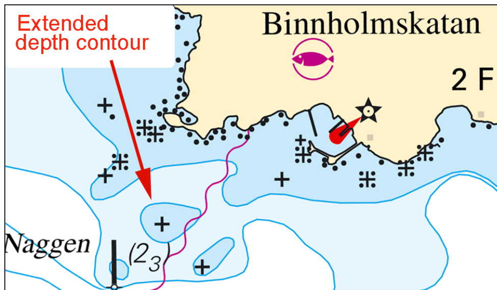
Uttökad djupkurva, Naggen
