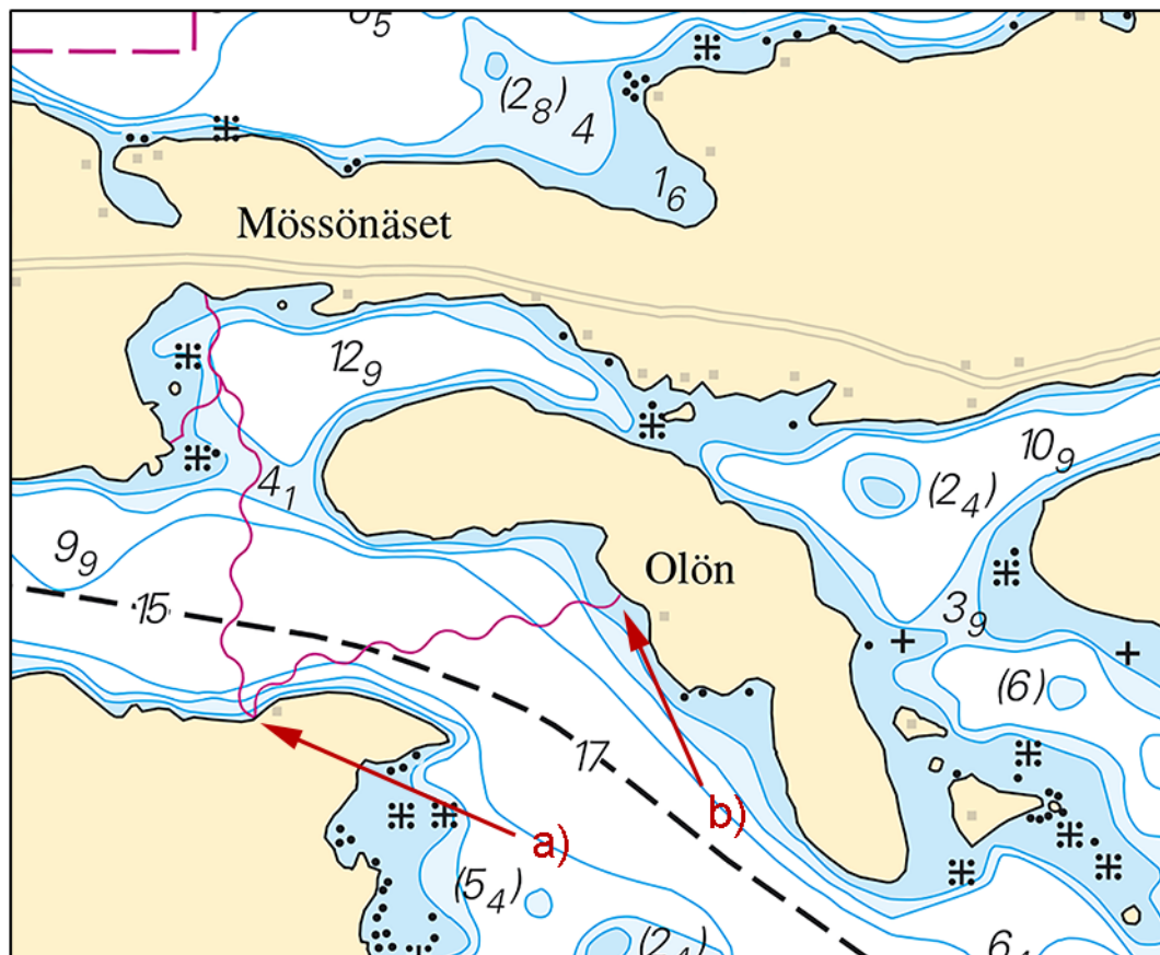
Njutångersfjärden. Kabel
