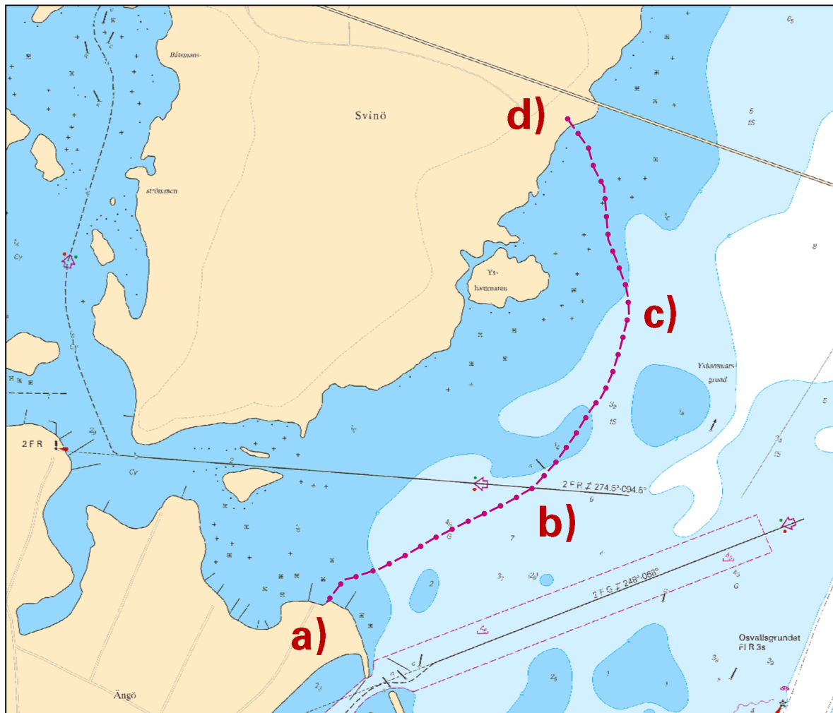
Rörledning Ängö - Svinö
