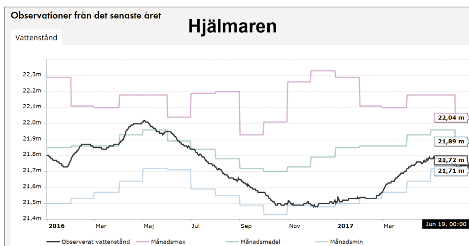
Diagram över vattenståndet i Hjälmaren under senaste året
