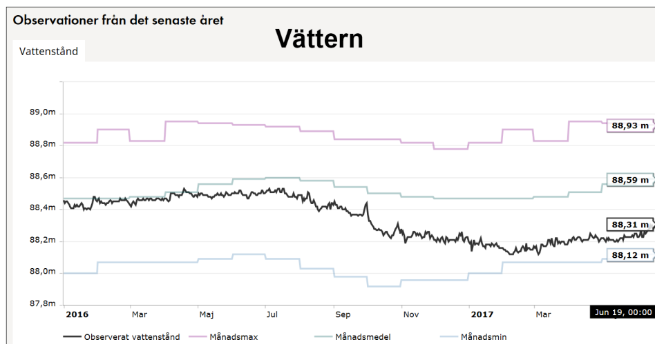
Diagram över vattenståndet i Vättern under senaste året
